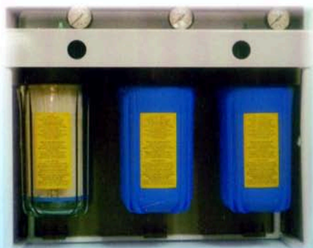
PW-H2濾心裝置圖
